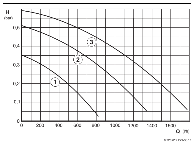
Fig. 34 Curve caratteristiche delle pompe con Logamax U052-24/28
